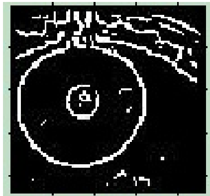
Fig.4 Edge Image
