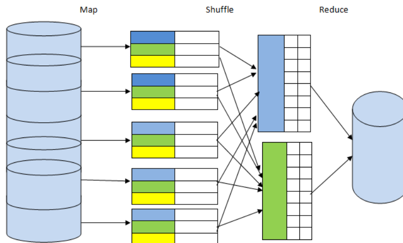
Fig: MapReduce
